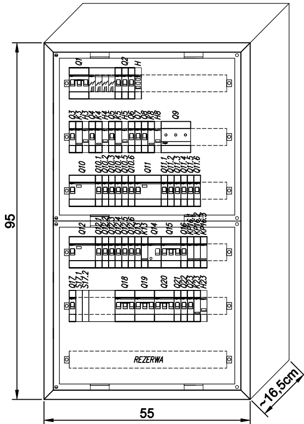
TABLICA HALI – TH WIDOK Z OTWARTYMI DRZWIAMI
