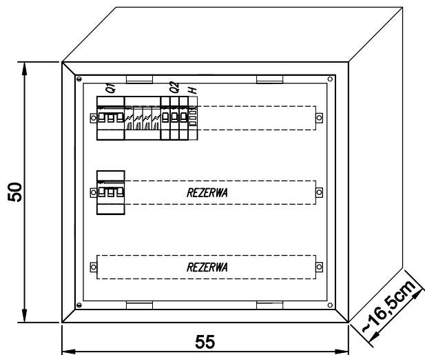
TABLICA POŻAROWA – TPOŻ WIDOK Z OTWARTYMI DRZWIAMI
